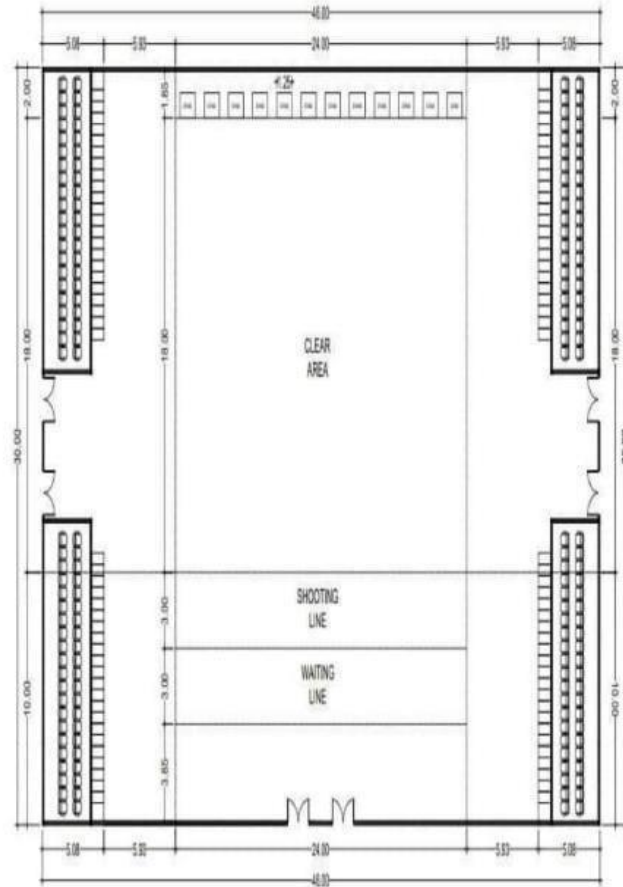
DENAH LANTAI SKALA 1:150
